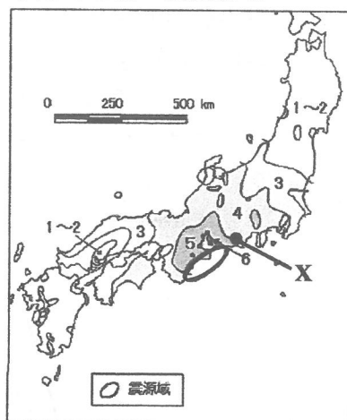
東南海地震の震度分布
