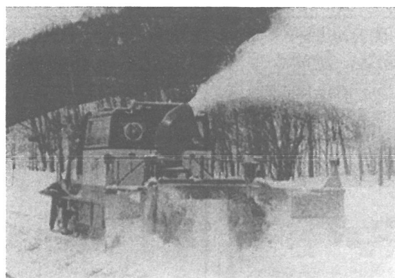
【資料 2】JR 北海道で活躍する機械の例
