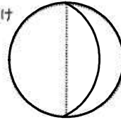
月食
