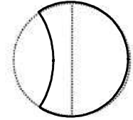
月食
