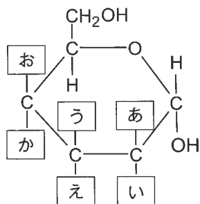
グルコース（ブドウ糖）
