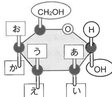
グルコースを立体的に表した図
