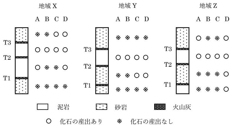
図2 地域X、Y、Zの地下の岩石のようす
