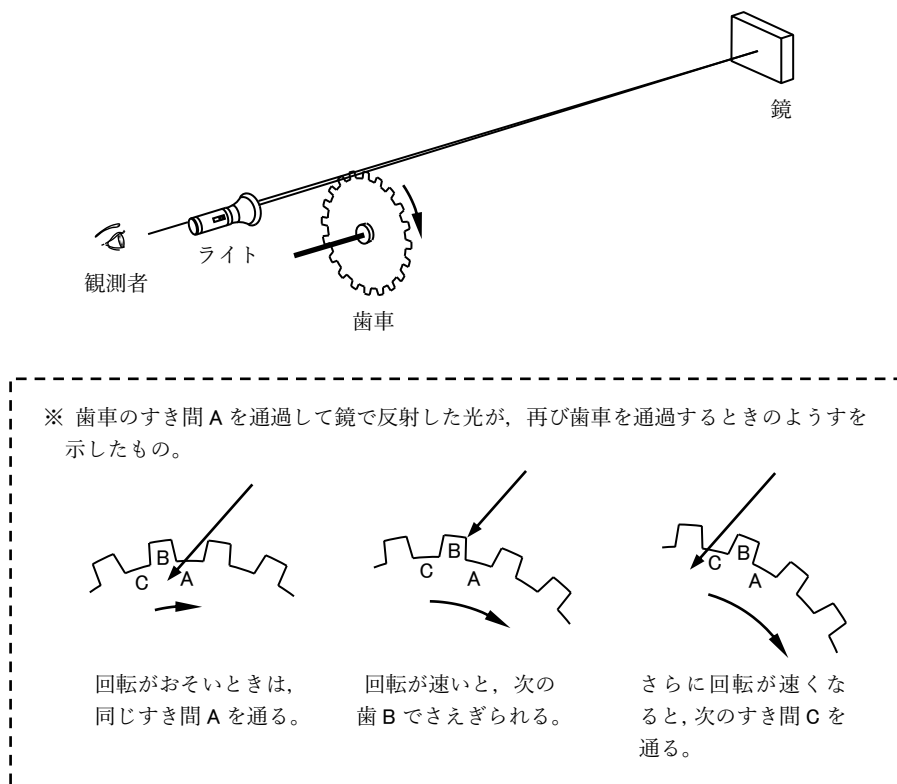
図1 フィゾーの実験装置
