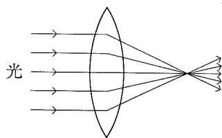
図6 凸レンズを通る光を横から見た図
