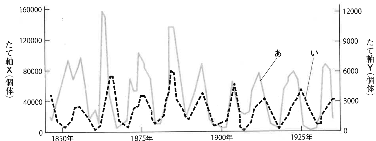
図3 カンジキウサギとカナダオオヤマネコの個体数の変動
