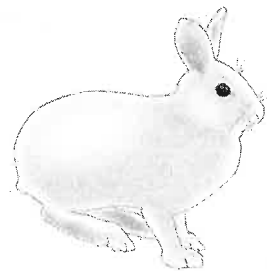
図1 カンジキウサギ
