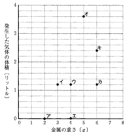
図2 じゅうぶんな量の水酸化ナトリウム水溶液を加えたときの反応
