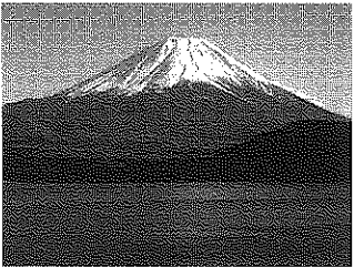
ア (富士山)
