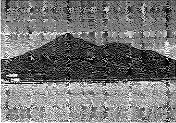
ウ (磐梯山)
