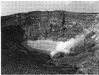
イ (阿蘇山)
