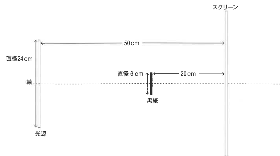
図3 実験1の断面図
