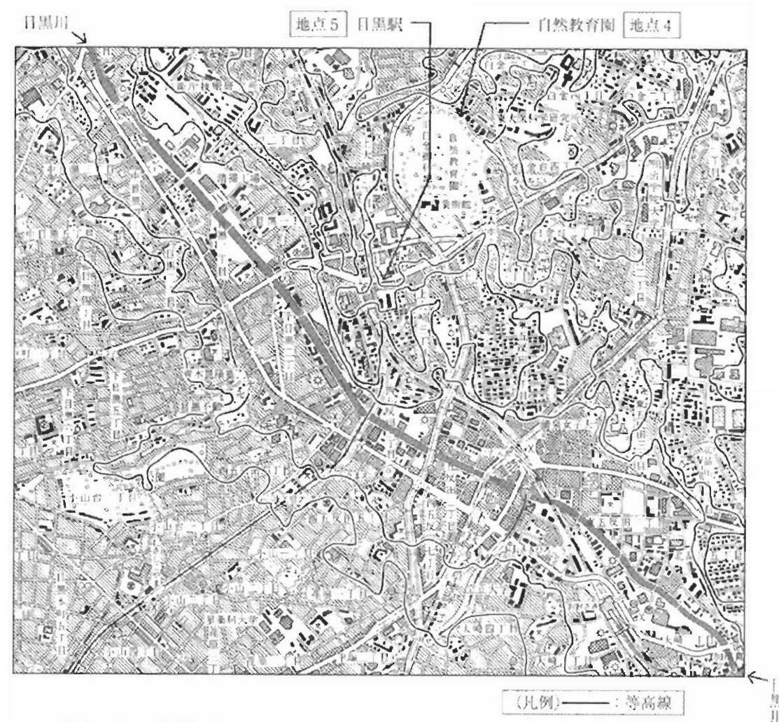
図4 地点4 から 地点5 までの周辺地図 (国土地理院発行 25000分の1地形図「東京西南部」を基に作成)
