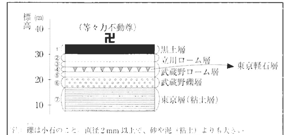
図6 等々力溪谷の断面スケッチ
