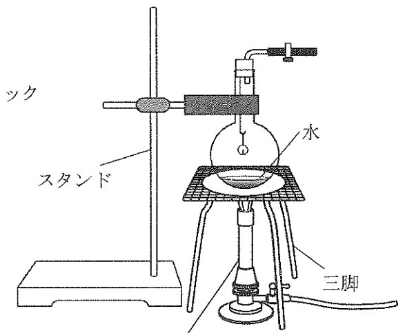
ガスバーナー 図 2
