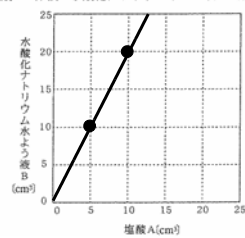
塩酸Aの体積と水酸化ナトリウム水よう液Bの体積の関係
