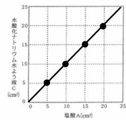
塩酸Aの体積と水酸化ナトリウム水よう液Cの体積の関係
