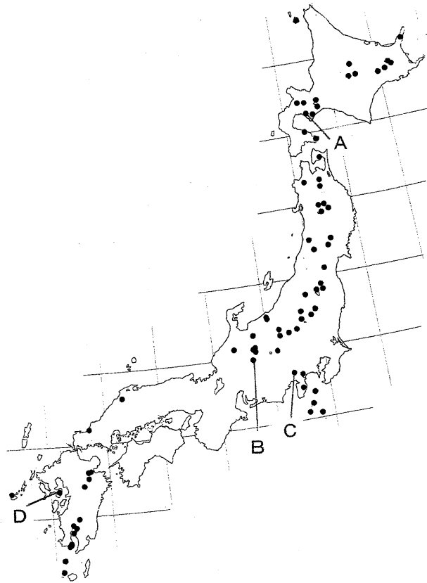
日本の主な活火山の分布 (一部省略)
