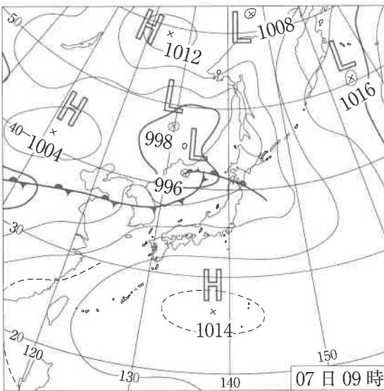
<天気図 C>
