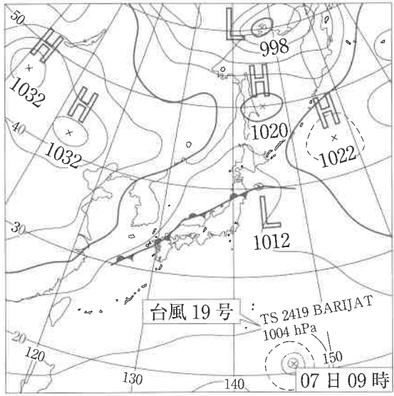
<天気図 B>
