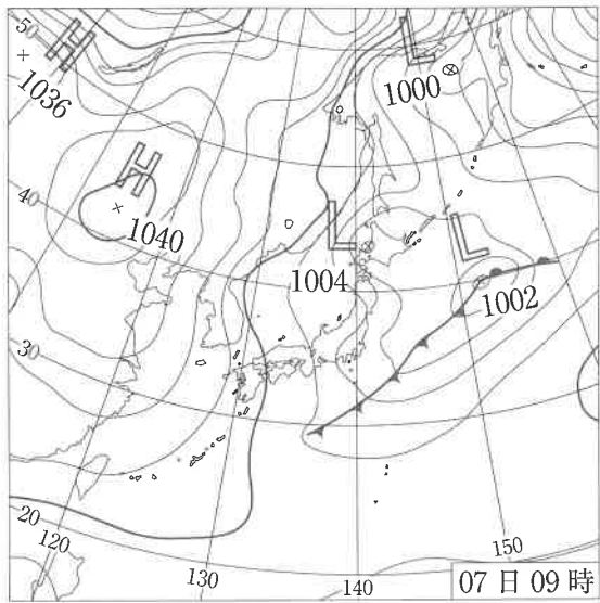
<天気図 A>
