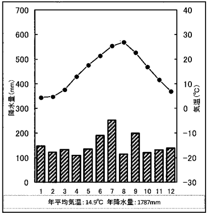
松江市の雨温図
