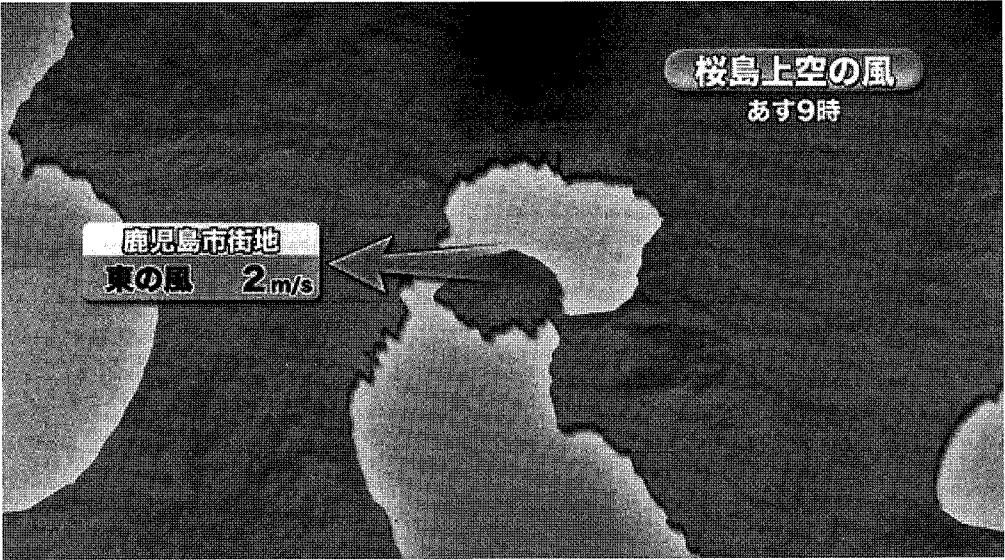
鹿児島テレビホームページ ニュース・天気より引用。 http://www.kts-tv.co.jp/tenki/sakurajima/index.php
