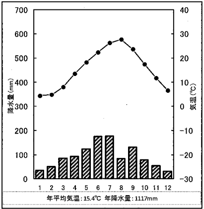
福山市の雨温図
