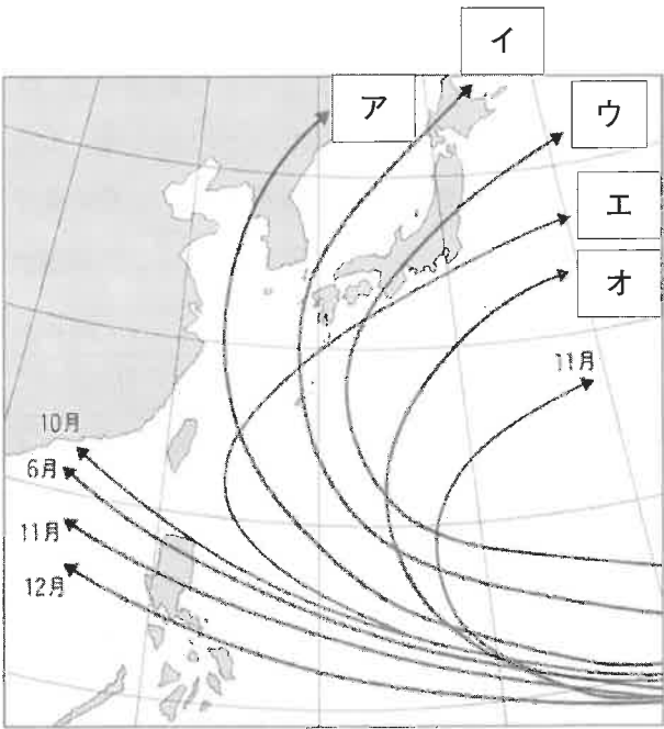
図3 日本にやってくる台風の月別平均進路 (日本気象協会)
