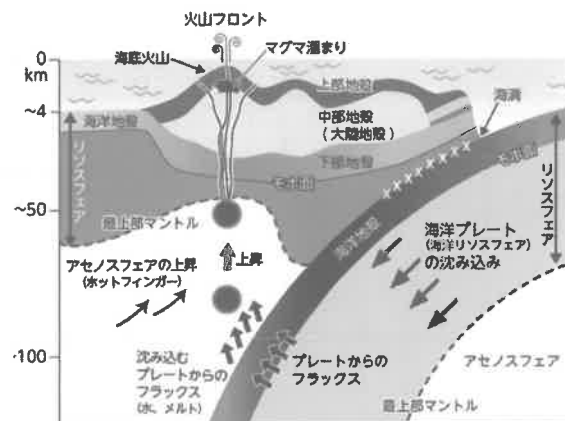
図 火山フロントの形成 伊豆小笠原弧の例
